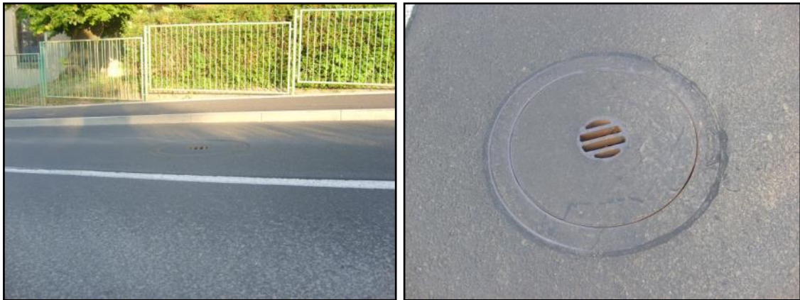
Abb. 34 Lärmarme Schachteindeckung (Beispiel Dresden)
